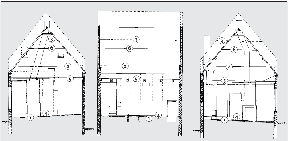
Afb. 5. Doorsnede door het huis, met bouwsporen in de muren. 1, 2 en 3: niveaus van begane grond, zolder en vliering van het oudste huis; 4, 5 en 6 idem van het 17de-eeuwse (huidige) huis; situatie 1992. Tekening: W. Brouwer.
