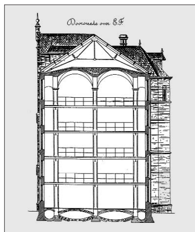
Afb. 7. Dwarsdoorsnede van het depotgebouw van het archiefgebouw.
