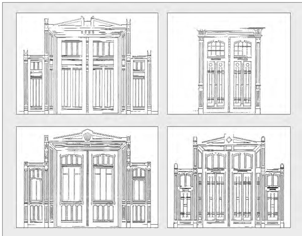
Afb. 5. Overzicht van vier deurpartijen van stoomtimmerfabriek Zeldenrust, 1906. Uit: catalogus van J. Timmer te Helpman bij Groningen, collectie M&M.
