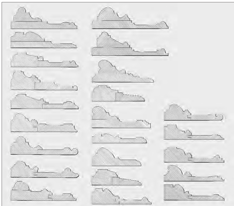
Afb. 4. Overzicht van deurlijstprofielen van stoomtimmerfabriek Zeldenrust, 1906. Uit: catalogus van J. Timmer te Helpman bij Groningen, collectie M&M.
