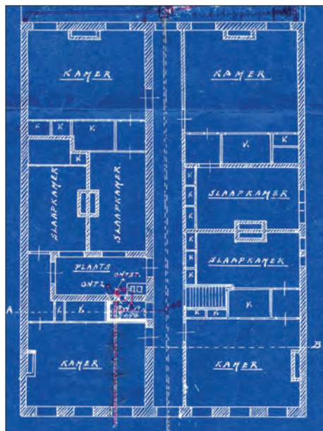
Afb. 10. Plattegrondtekening uit 1927. Tekening: bouwdoossier Dienst RO/EZ.
