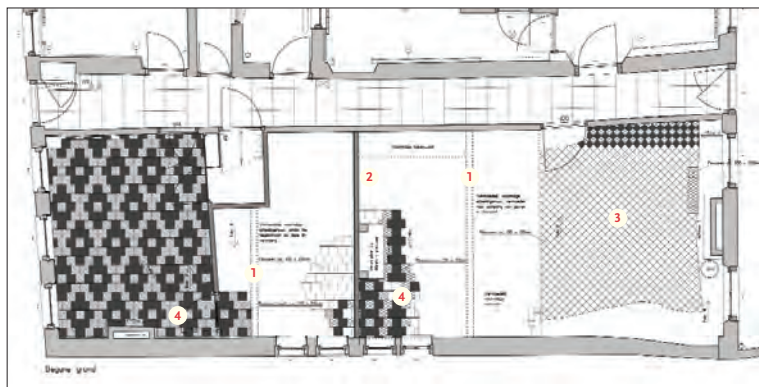
Afb. 6. Opmetingstekening uit 2007 waarop diverse bouwsporen zijn vastgelegd: 1: plaats van muren die horen bij de 17e- en 18e-eeuwse indeling; 2: later aangebrachte muur (19e eeuw?); de haardplaats tegen deze muur is over de 18e-eeuwse vloer aangebracht; 3: de 17e-eeuwse vloer; hierop lagen de restanten van de 18e-eeuwse plavuizenvloer, gelegd in een ruitpatroon zoals in de voorste kamer (links op de tekening); 4: 18e-eeuwse plavuizenvloeren. Tekening: Daniël van Huizen, collectie Holstein Restauratie Architectuur.
